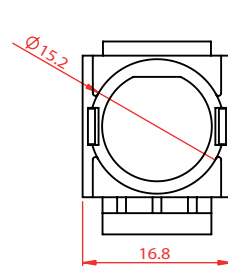
剖面圖 A-A 比例 2 : 1
